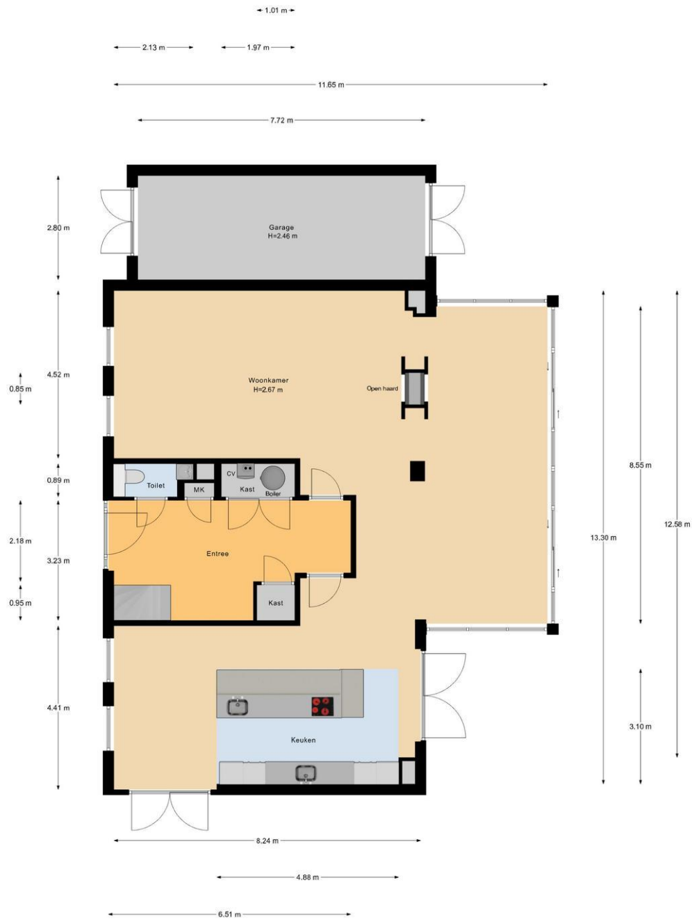
Begane Grond
