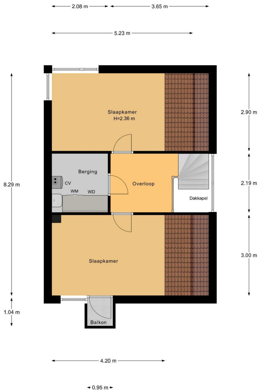
2e Verdieping
