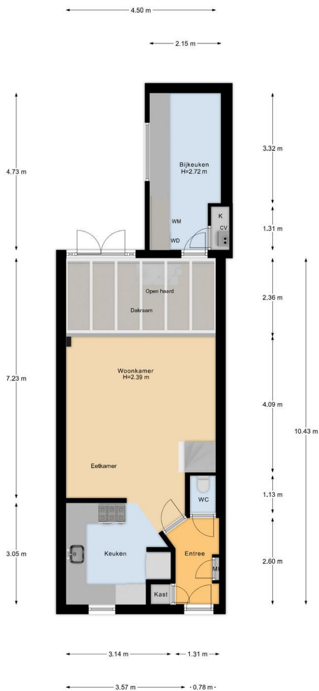
Begane Grond
