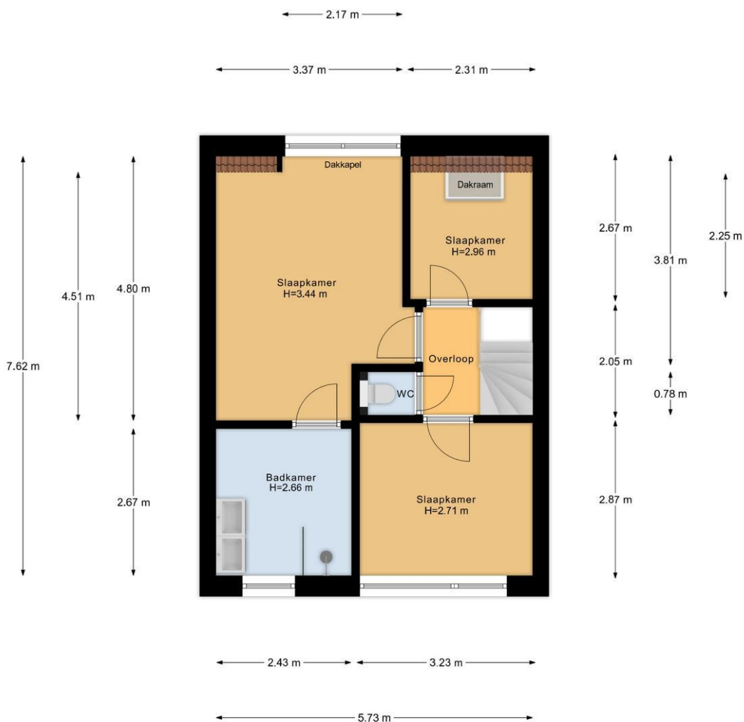
1e Verdieping
