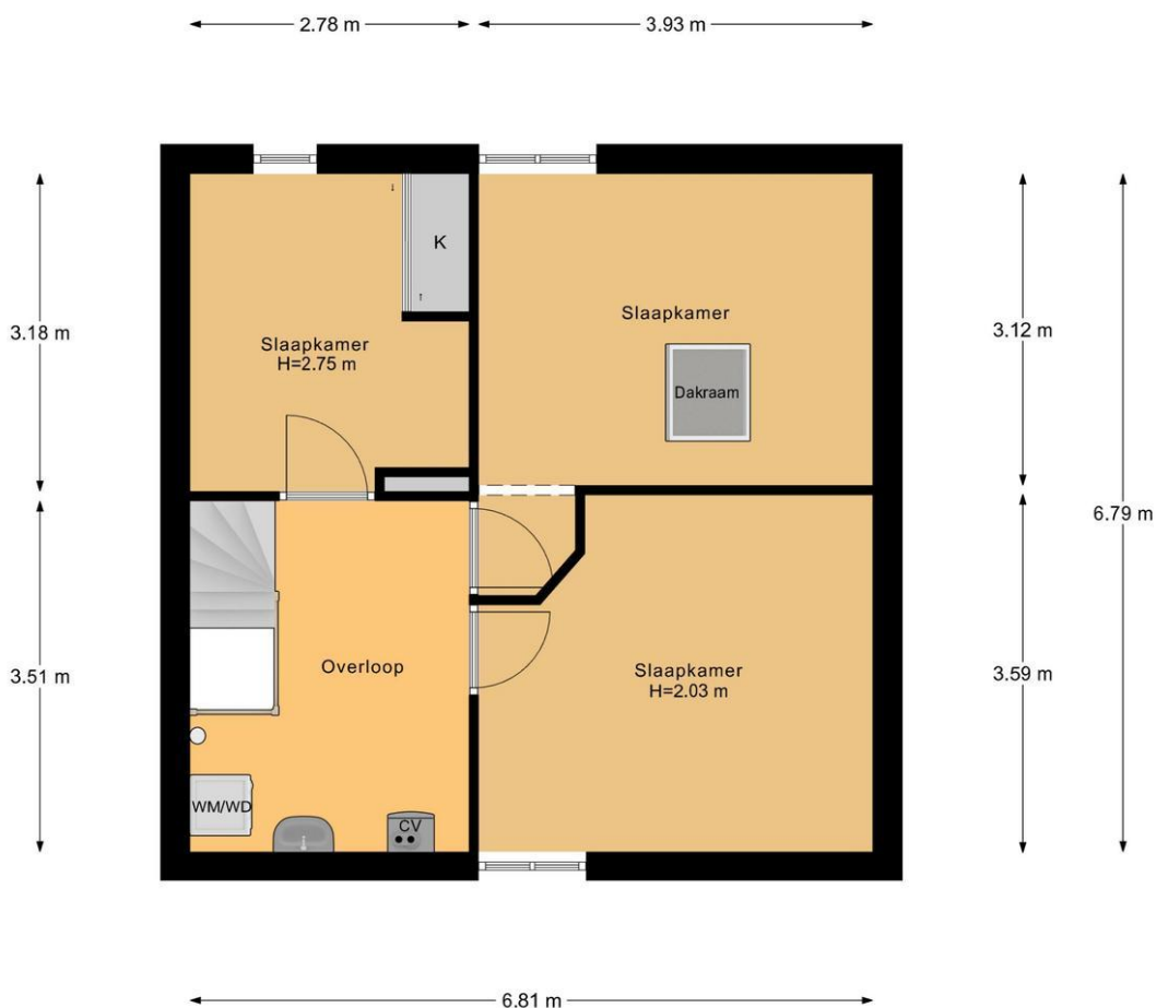
2e Verdieping
