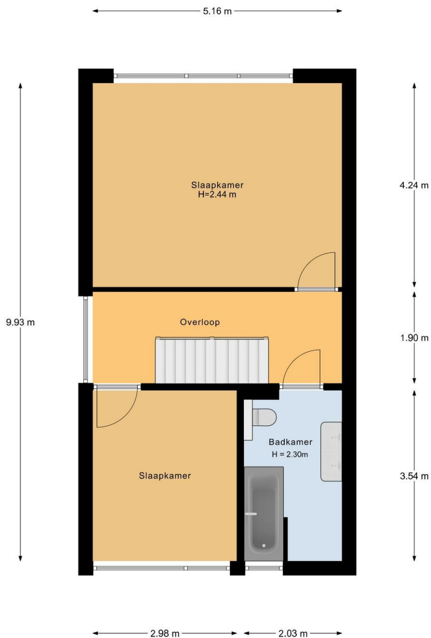
1e Verdieping
