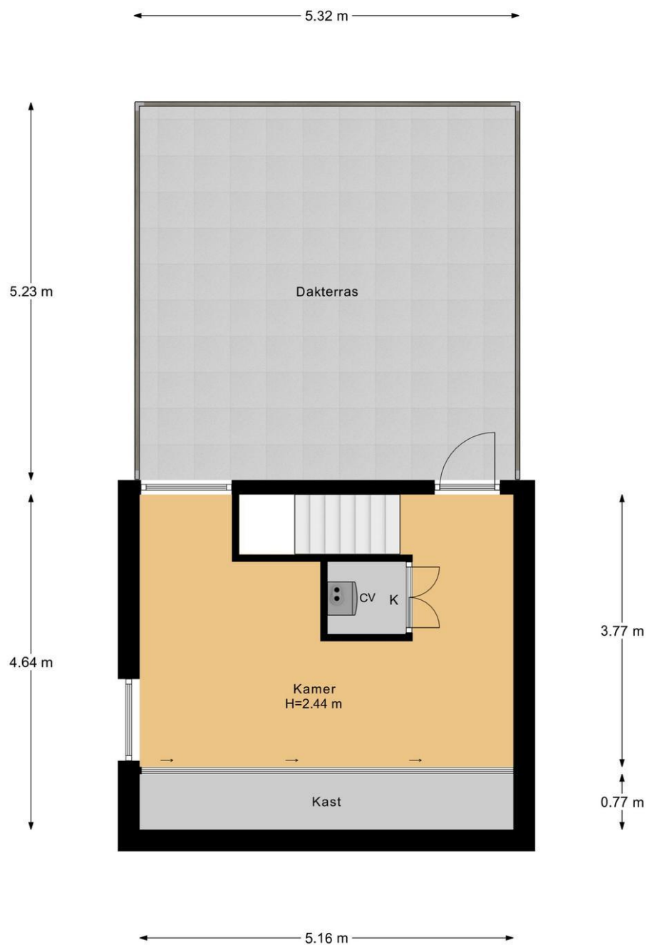
2e Verdieping
