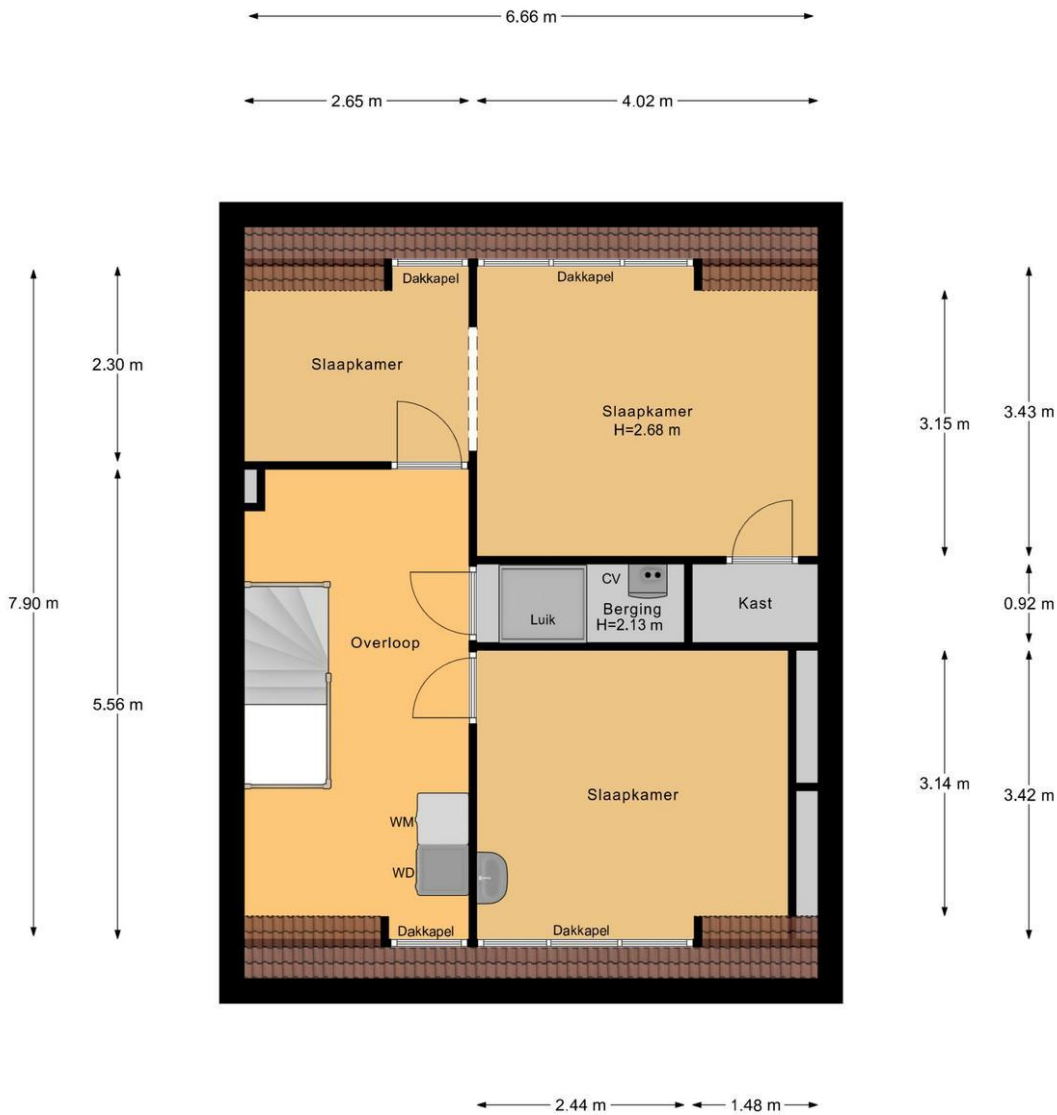
2e Verdieping
