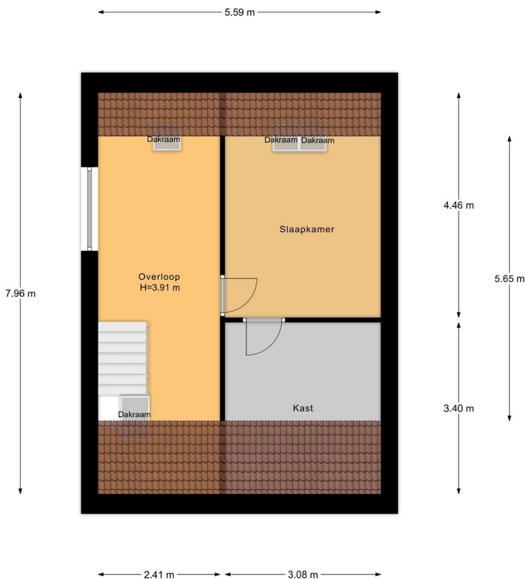
2e Verdieping
