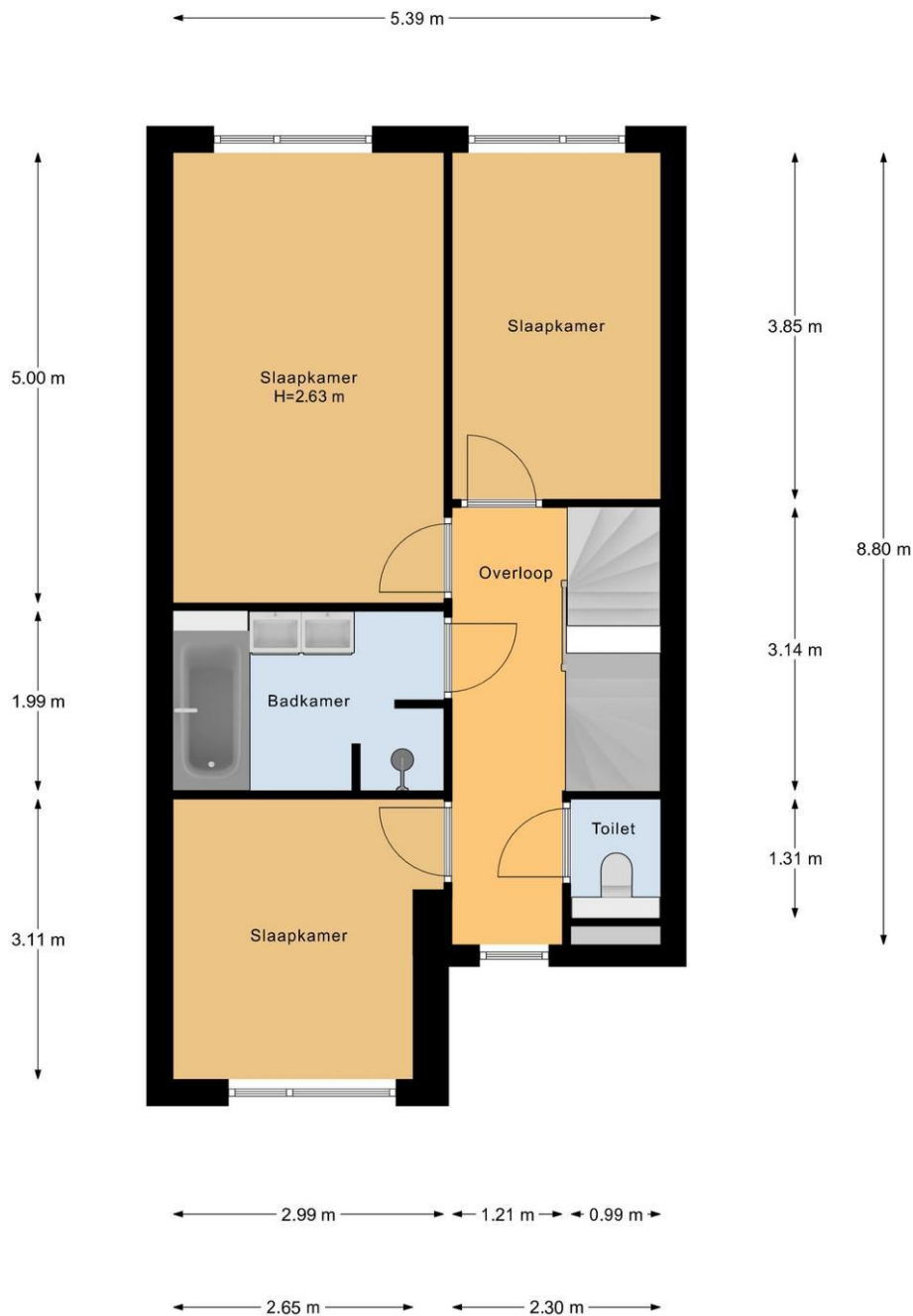
1e Verdieping
