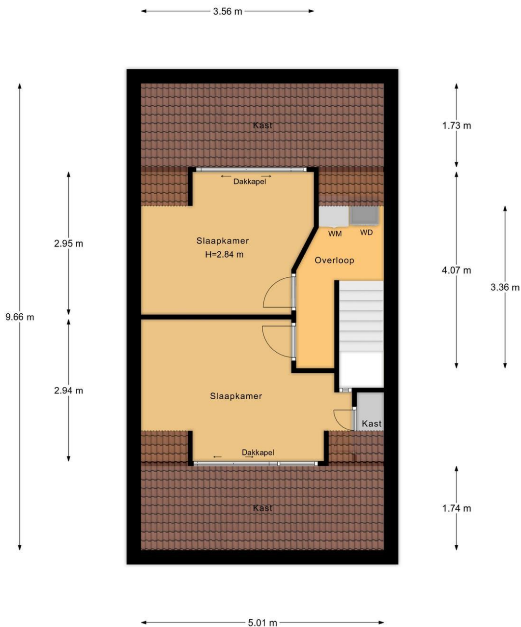
2e Verdieping
