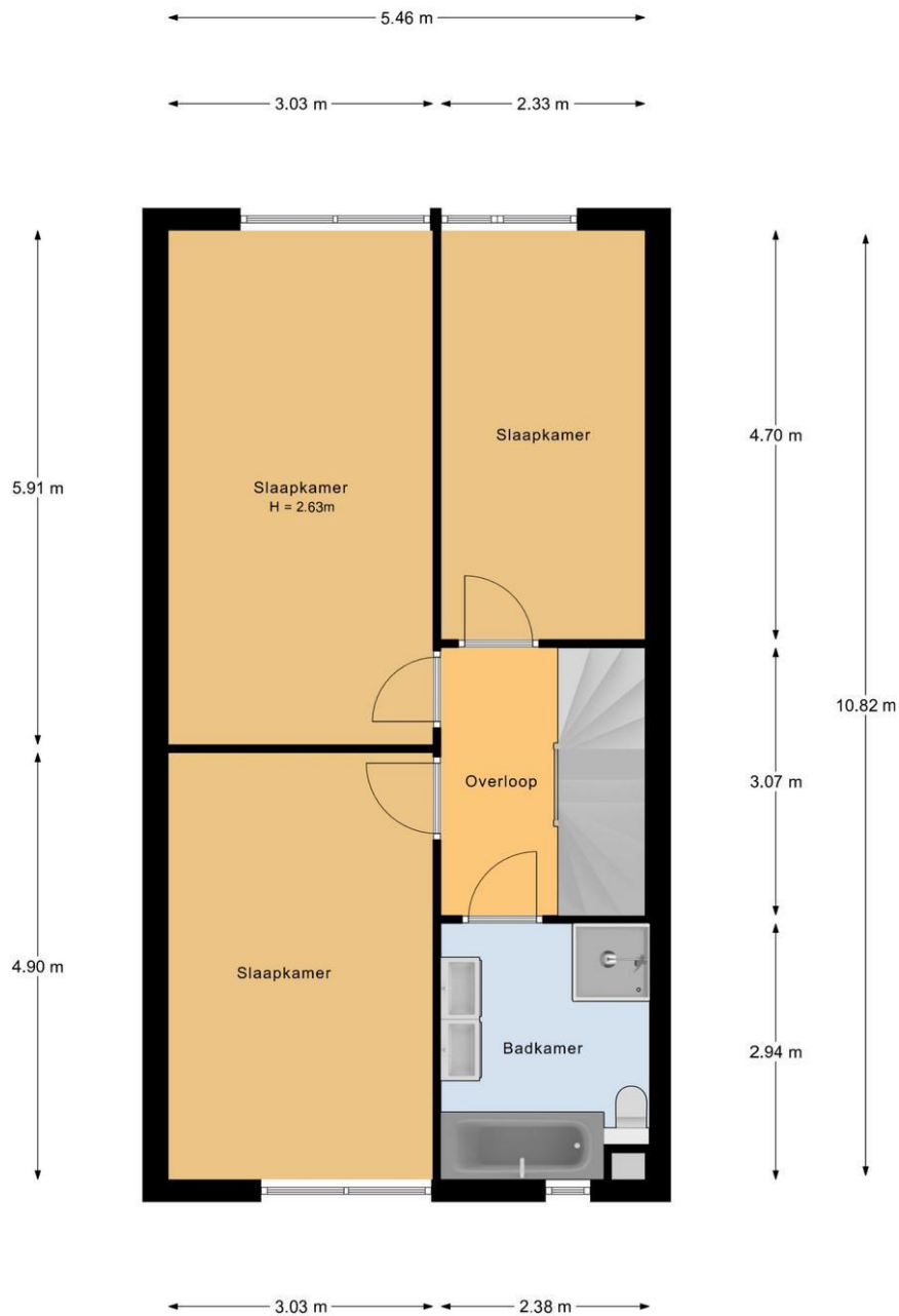
1e Verdieping
