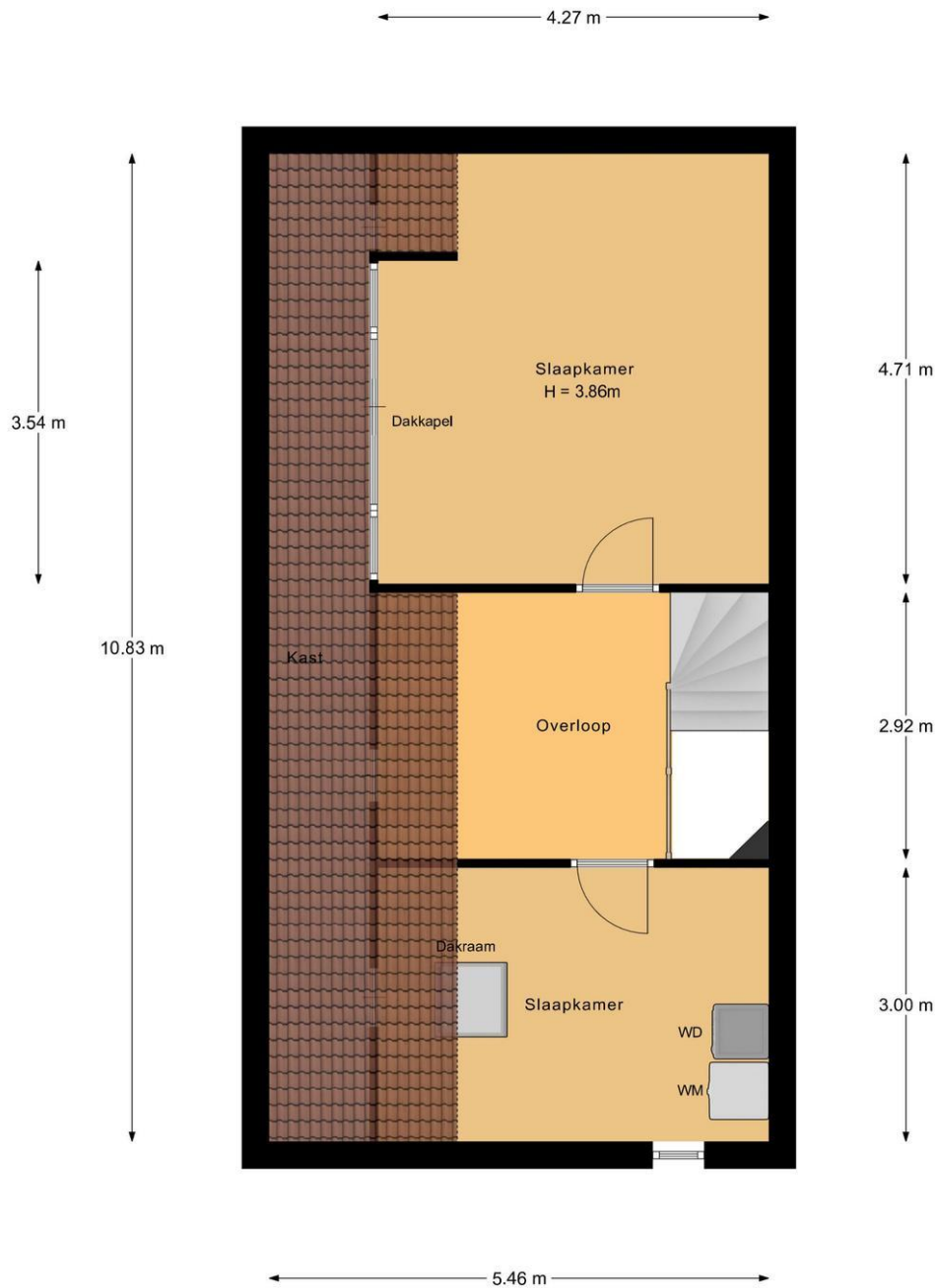
2e Verdieping
