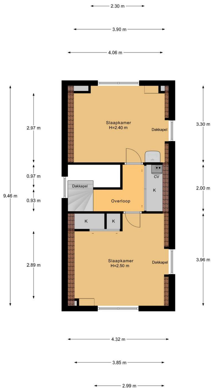
1e Verdieping
