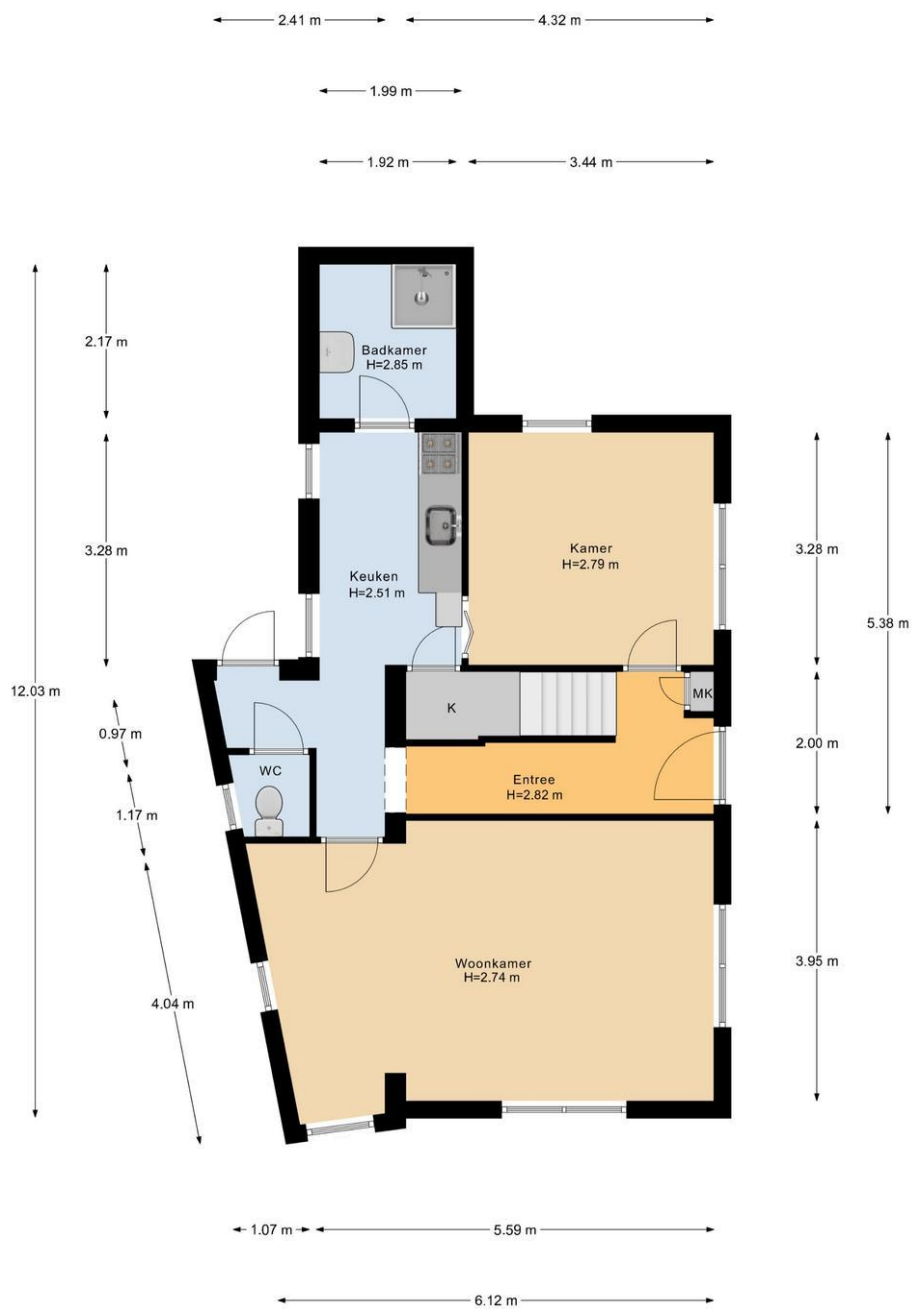
Begane Grond
