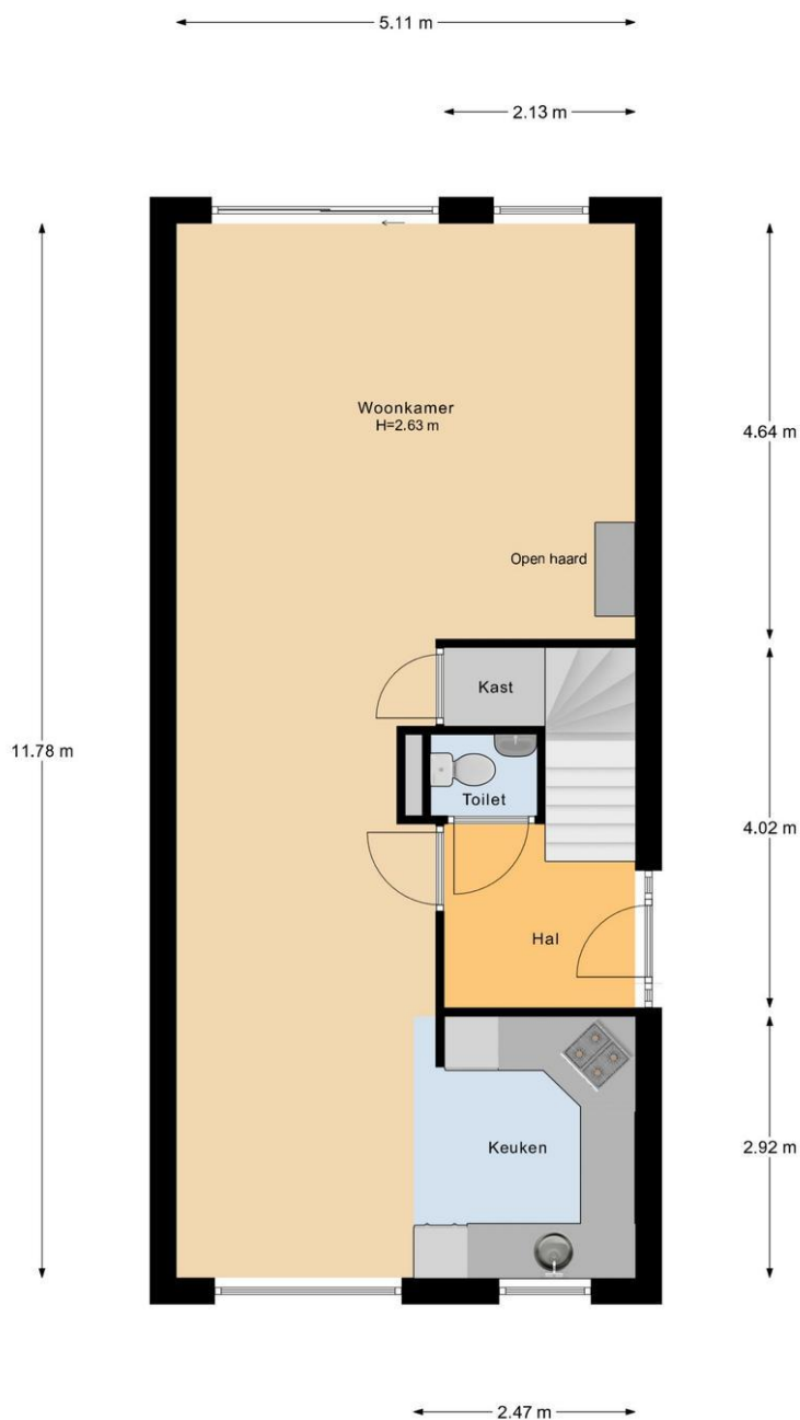
Begane Grond
